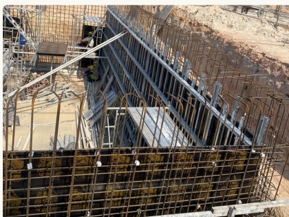
Cốt thép, ván khuôn tường BTCT
